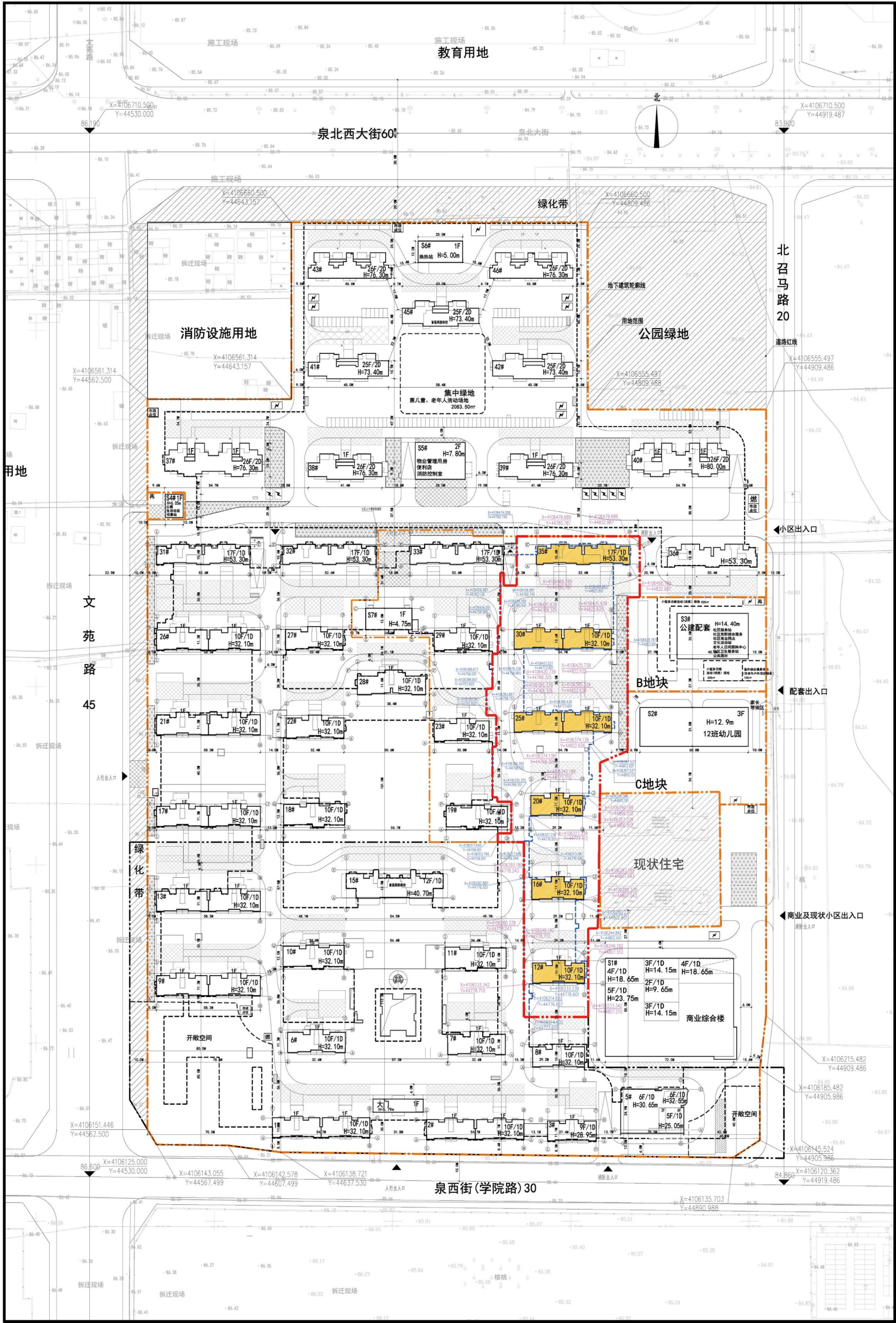
放线定位图
